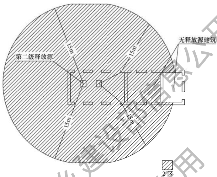
图 E.0.5 与具有第二级释放源的建筑物相邻，并采用不燃烧体实体墙隔开时，其爆炸危险区域和范围划分的最高浓度不超过其爆炸下限 10% 的区域；
